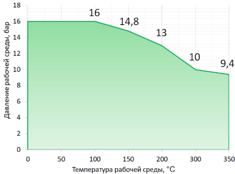
График зависимости температуры и давления рабочей среды
