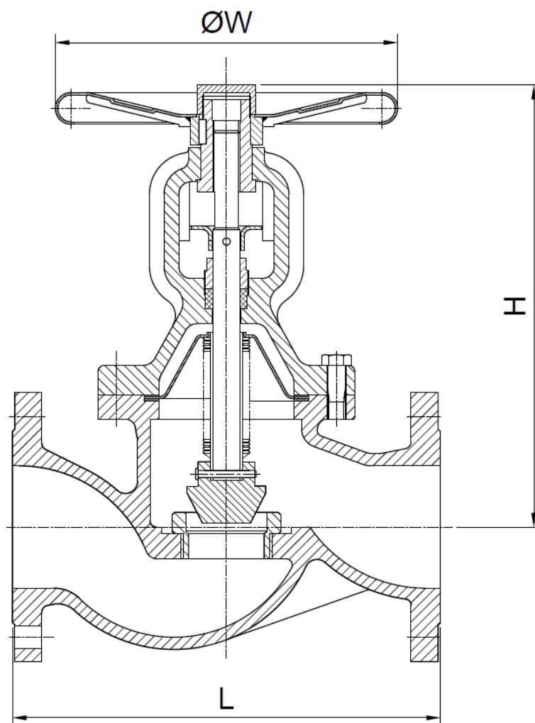
Рисунок 2. Основные массогабаритные характеристики клапана запорного с сильфонным уплотнением DN15-100 PN16
