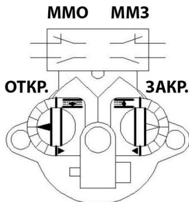
Рис.4. Блок моментных выключателей
