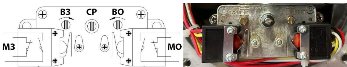
Рис. 3. Блок концевых выключателей
