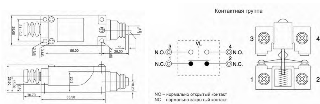
Размеры и схема контактной группы концевых выключателей
