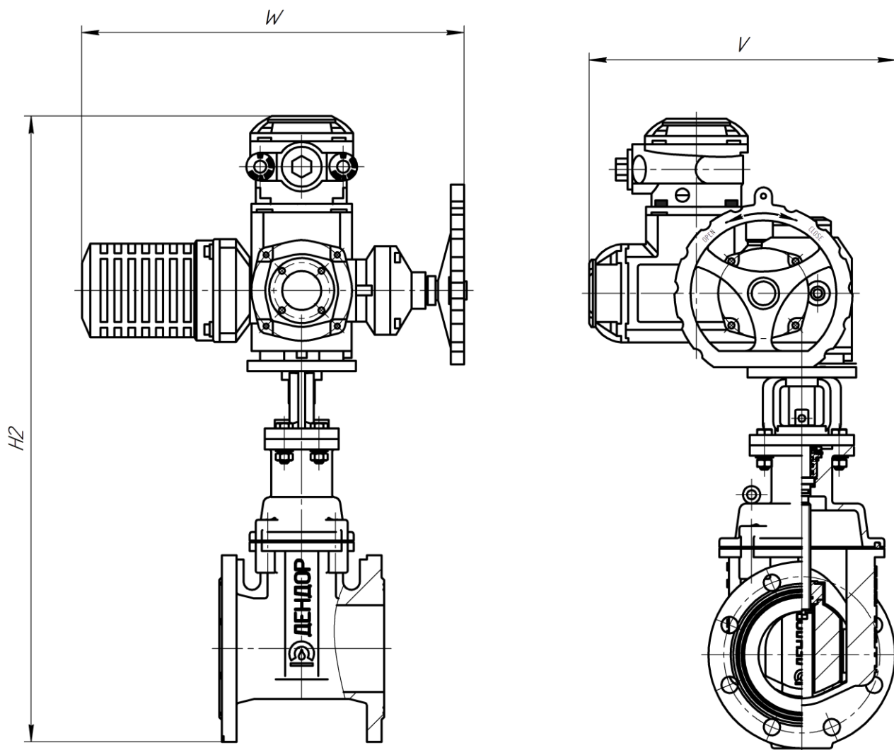
Рисунок 2. Задвижка с адаптером-переходом под ISO фланец и электроприводом MT903.A DN50-300
