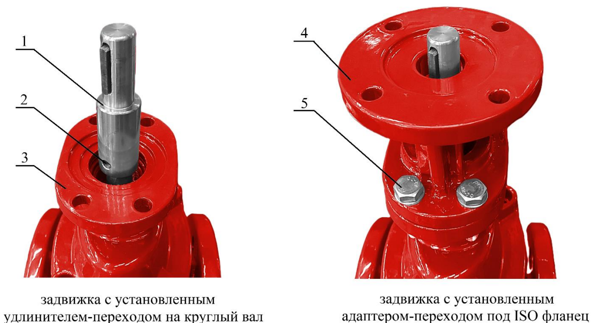
Рисунок. Монтаж адаптера-перехода под ISO фланец
