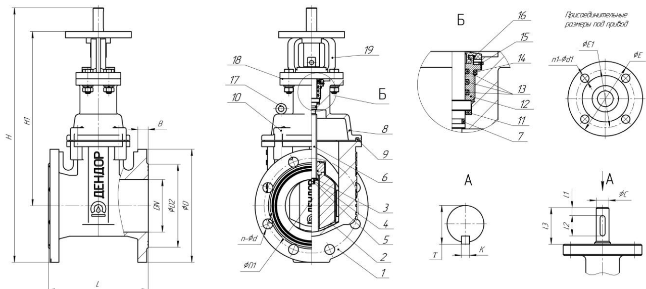
Рисунок 1. Задвижка с адаптером - переходом под ISO фланец DN50-300
