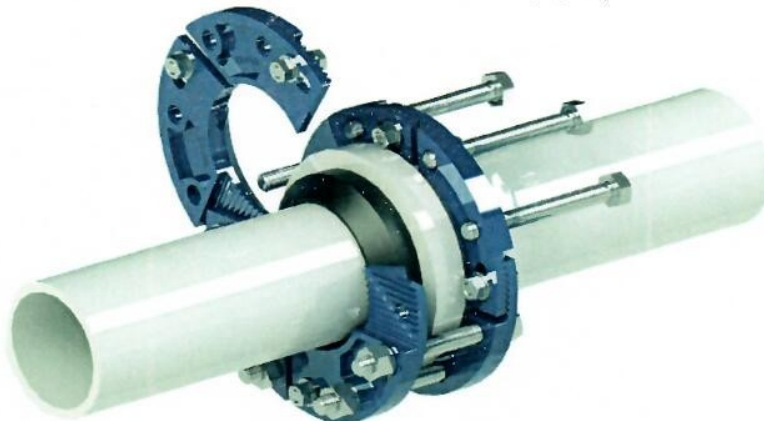
Рисунок 1 – Общий уплотнитель раструбный DENDOR тип RS-C17
