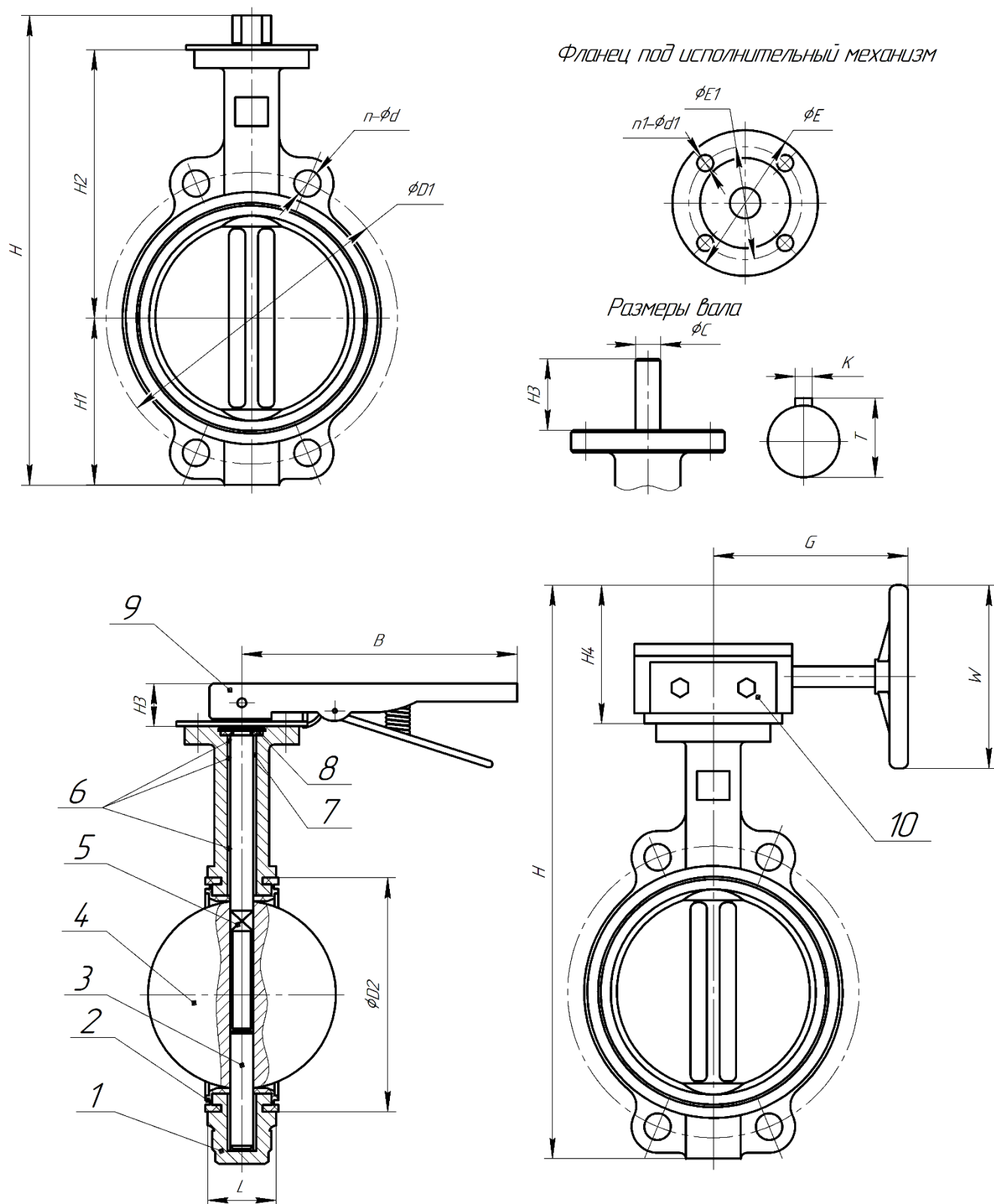
Рисунок 1. Затвор 017W.YS PN16 DN32-600 и 017W.ZS PN25 DN32-600
