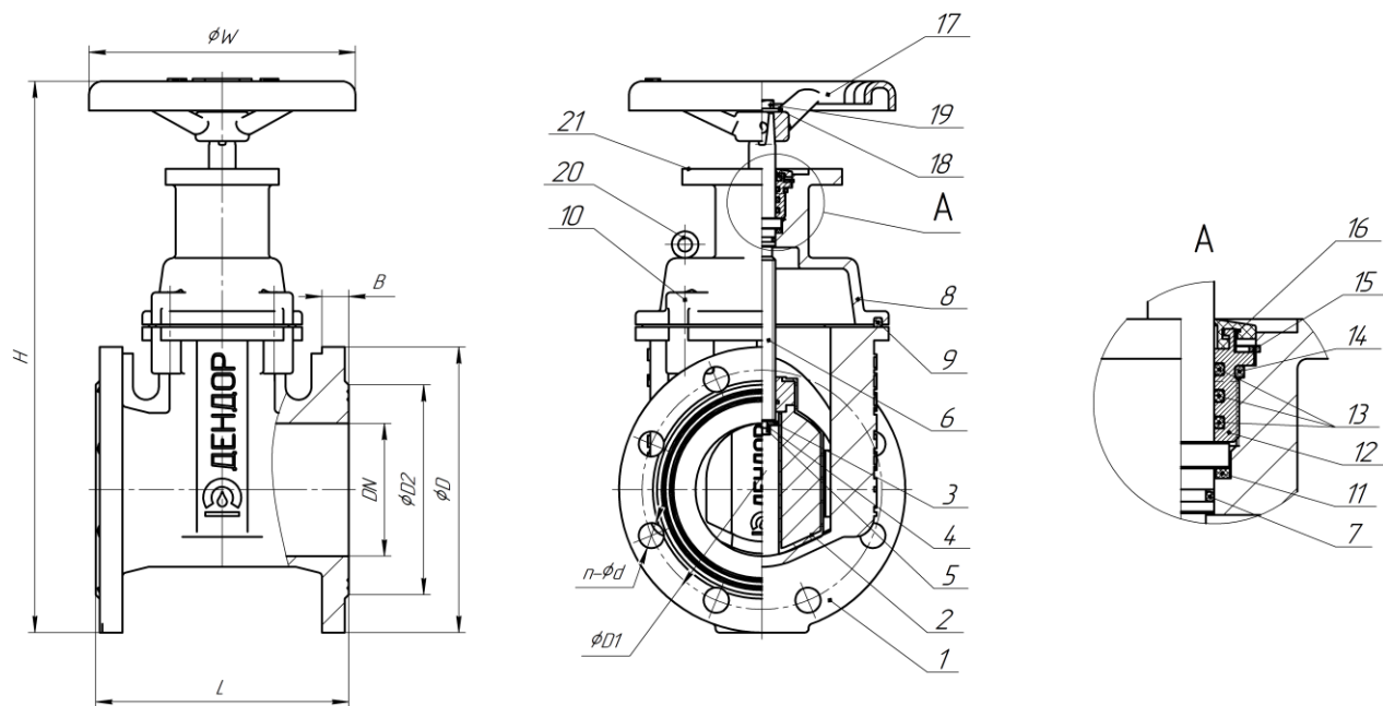
Рисунок 1. Задвижка с маховиком DN50-300
