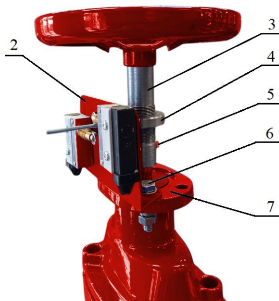
задвижка с установленным УКП
