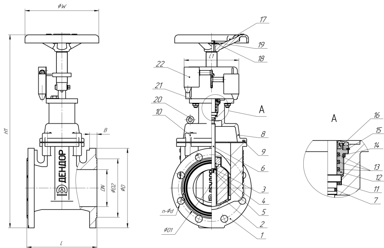
Рисунок 2. Задвижка с маховиком и УКП DN50-300
