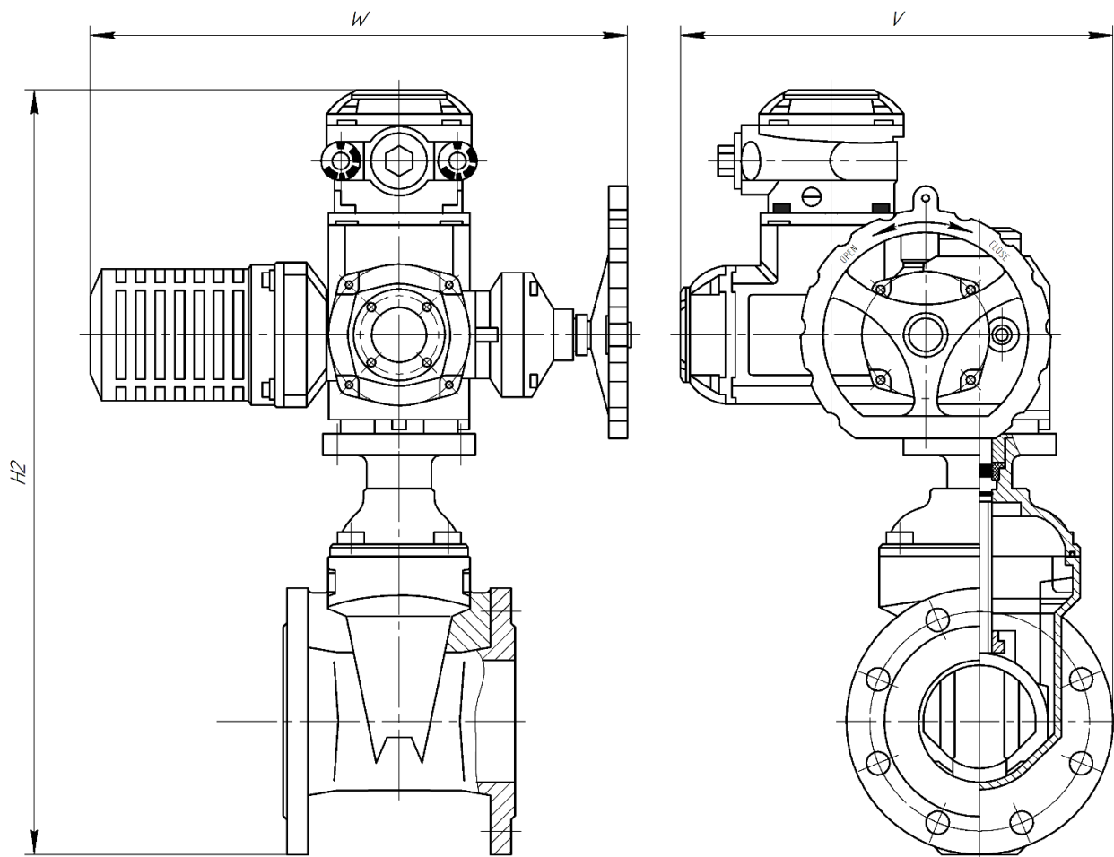
Рисунок 2. Задвижка с электроприводом тип MT903.A DN50-300
