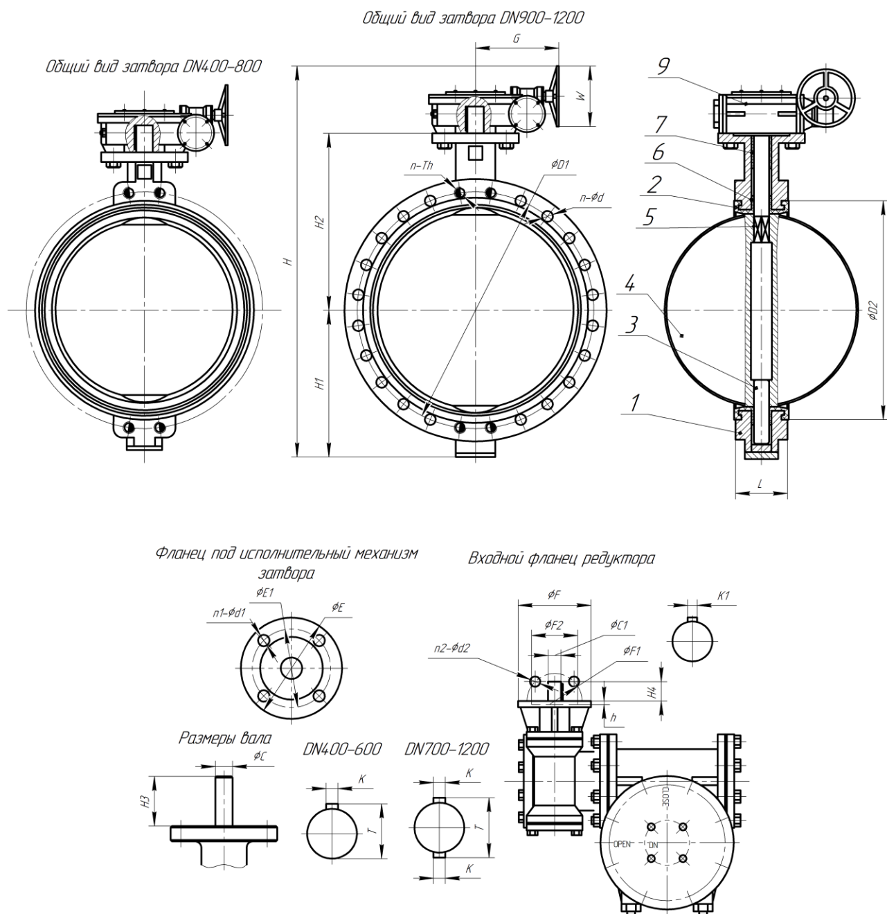
Рисунок 3. Затвор 017W.YS с редуктором DN400-1200
