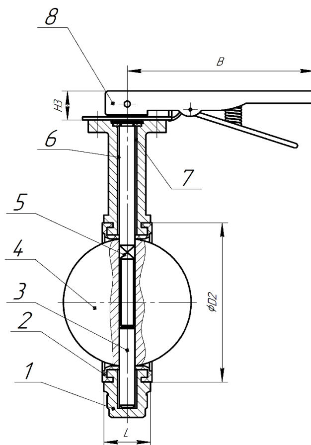
Рисунок 1. Затвор 017W.YS с рукояткой DN32-40
