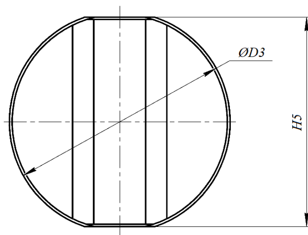
Рисунок 4. Диск затвора
