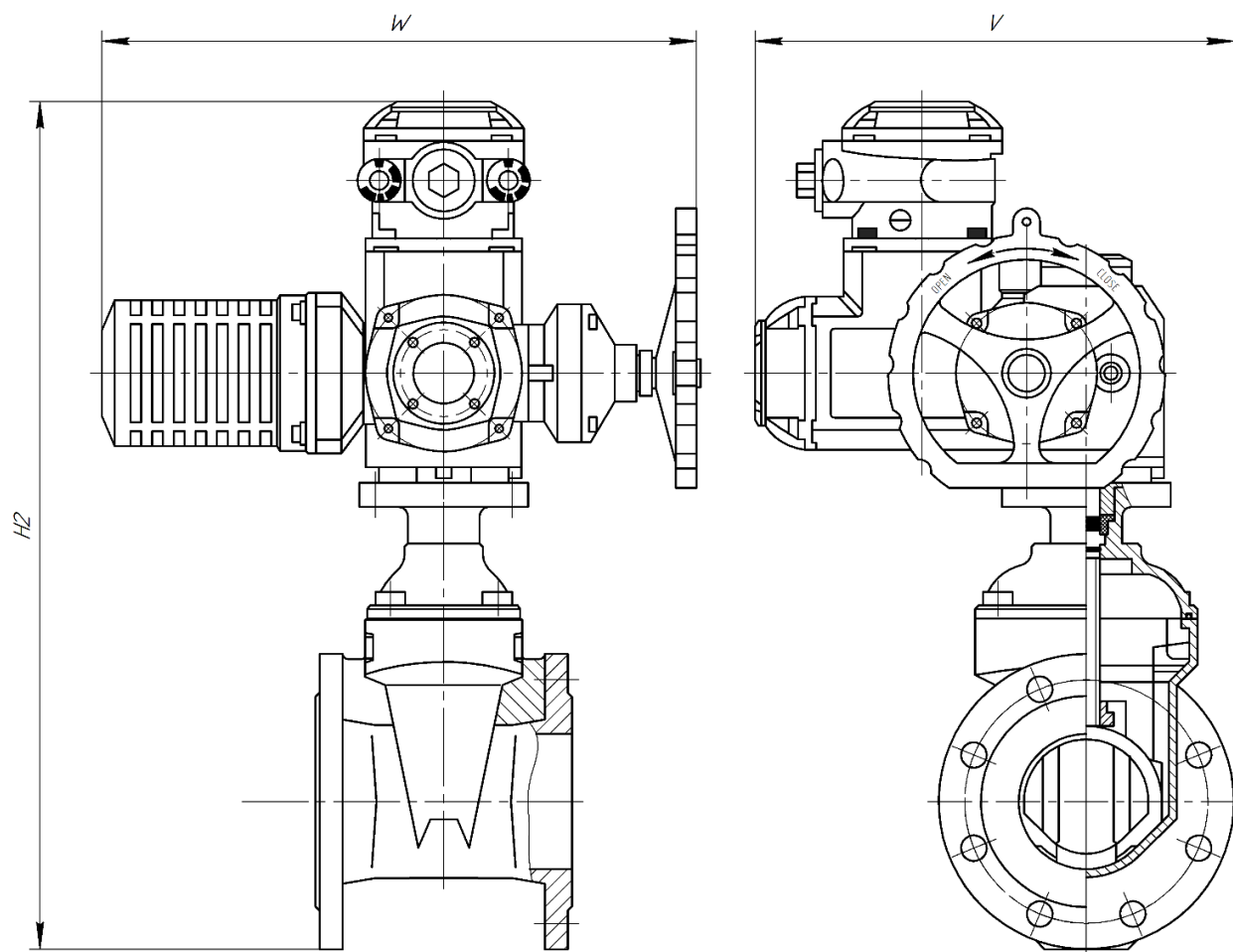
Рисунок 2. Задвижка 47GVA.Z с электроприводом тип MT903.A DN350-1200
