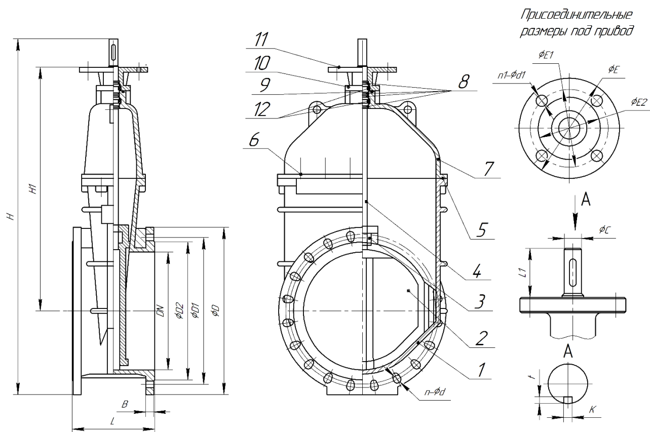
Рисунок 1. Задвижка 47GVA.Z без исполнительного механизма DN350-1200
